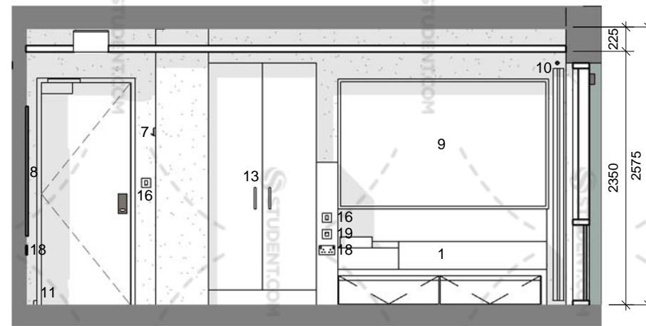
NTB6-W 1 : 50
