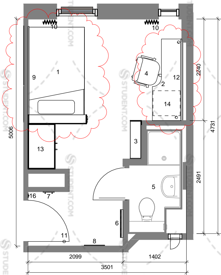
NTB6 - Layout Plan 1 : 50
